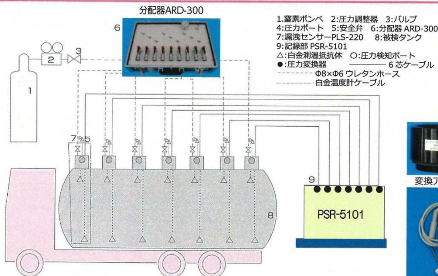
漏洩センサー取付例
